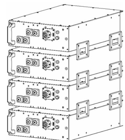
Montaje en bloque con abrazaderas
