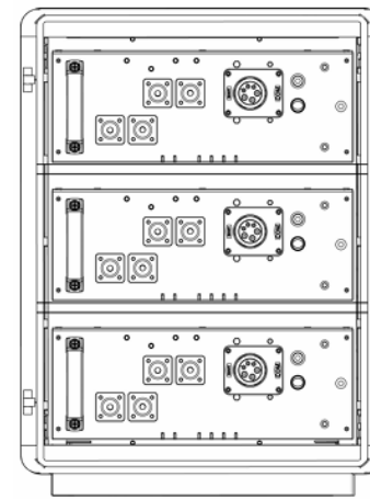
Instalación dentro de gabinete
